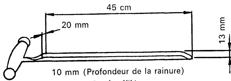
Fig. 1. Sonde effilée ouverte
