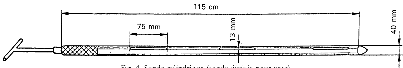
Fig. 4. Sonde cylindrique (sonde divisée pour vrac)
