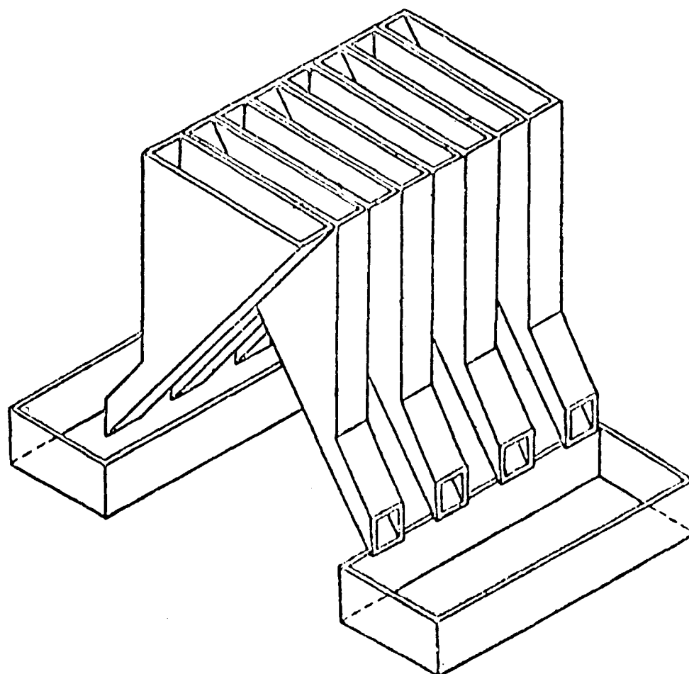
Fig. 9. Echantillonneur à multiples fentes
