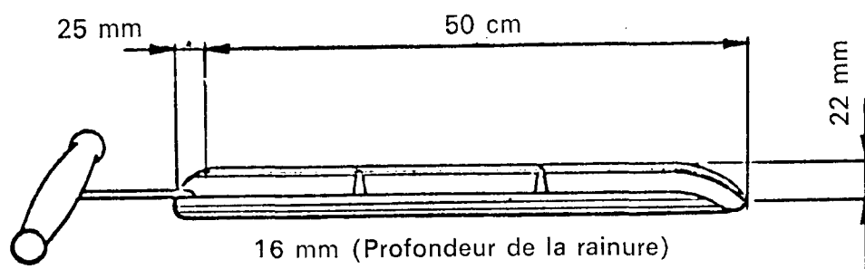
Fig. 3. Sonde effilée ouverte, divisée
