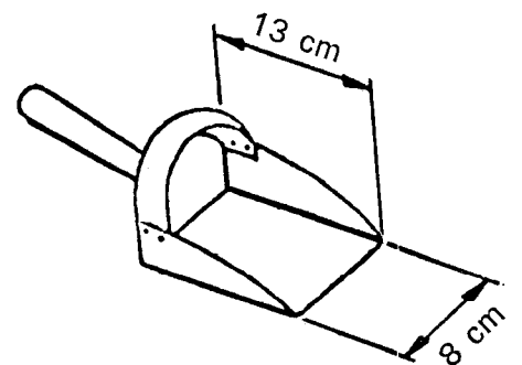
Fig. 2. Pelle à main
