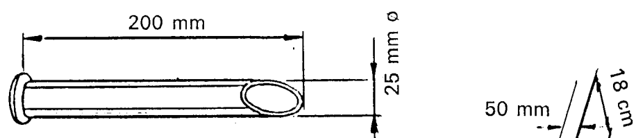
Fig. 5. Sonde spécialement conçue pour les sacs
